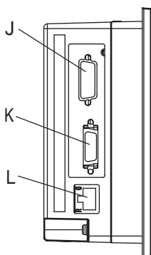
左側面図
