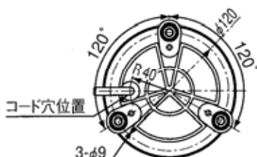
取付寸法
