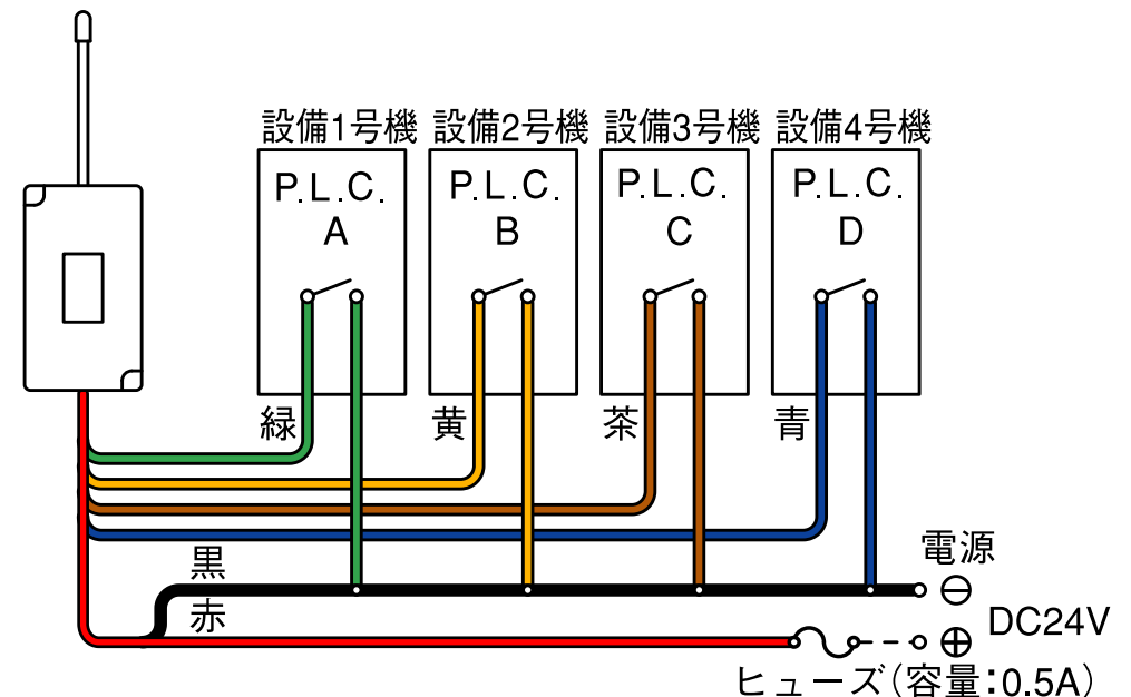
送信機 例2 (1台の送信機で設備4台に接続する時)
