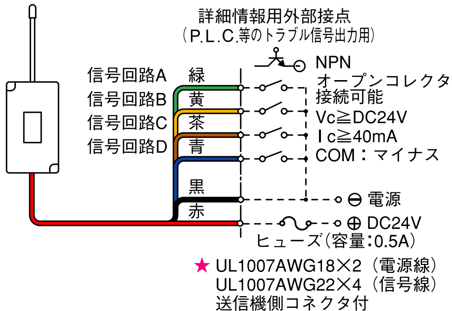
送信機 例1 (設備1台に対して4種類のトラブル内容識別を行なう時)
