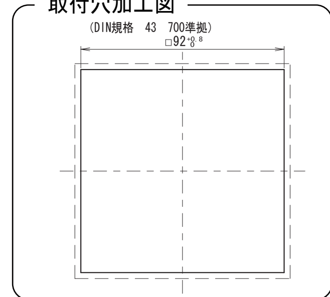
取付穴加工図
