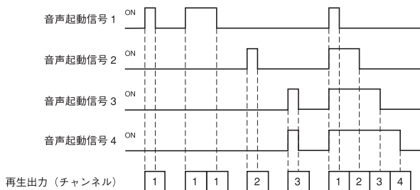
ビット入力タイムチャート
