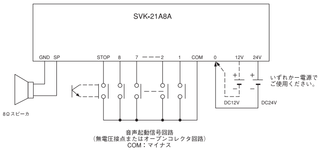
図8 結線例
