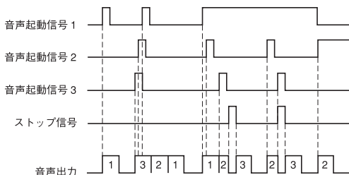
動作モードB タイムチャート
