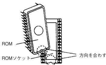
図9 音声ROMの方向
