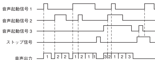
動作モードD タイムチャート
