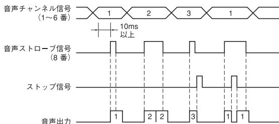
動作モードG タイムチャート
