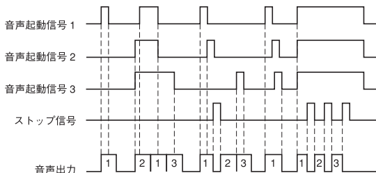
動作モードA タイムチャート
