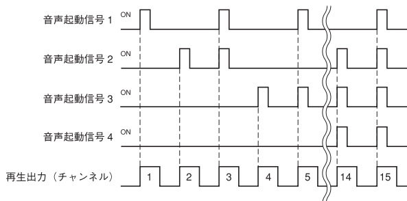
バイナリー入力タイムチャート
