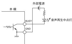
図6 BUSY (オープンコレクタ出力) 接続例
