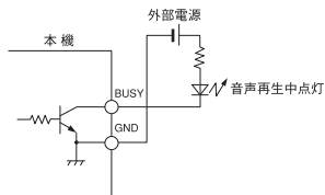
図2 BUSY (オープンコレクタ出力) 接続例
