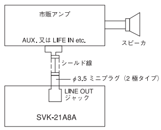
図7 LINE OUT使用例
