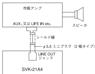
図3 LINE OUT使用例
