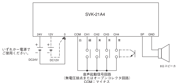
図4 結線例
