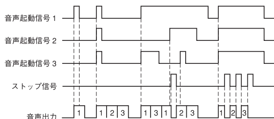
動作モードC タイムチャート
