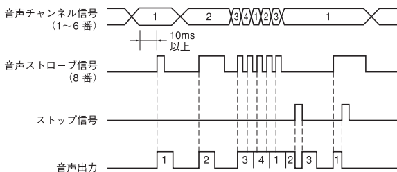
動作モードH タイムチャート
