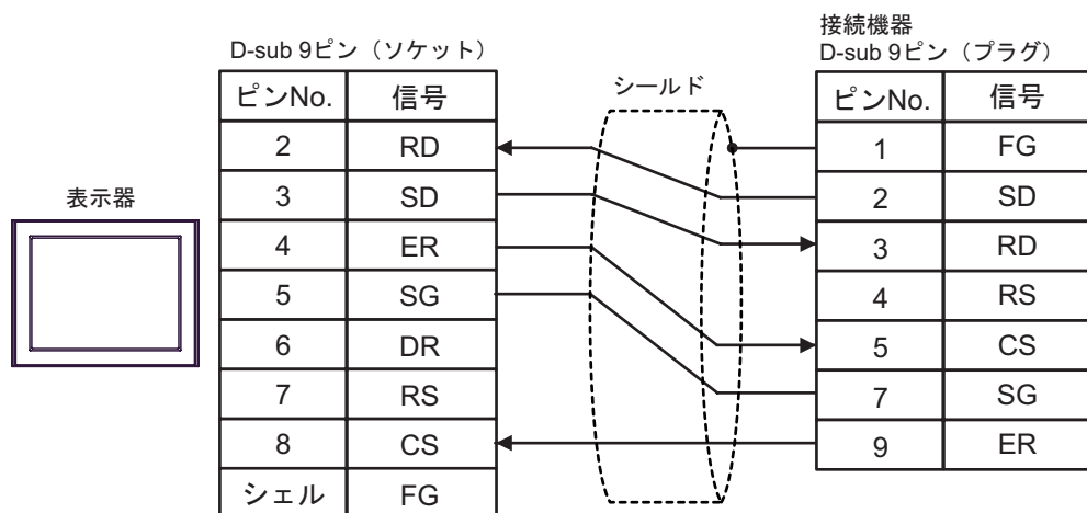
結線図 8
