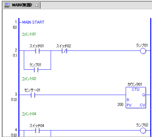
ラダー方式
