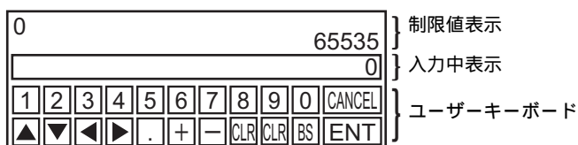
ユーザーキーボード + 入力中表示 + 制限値表示
