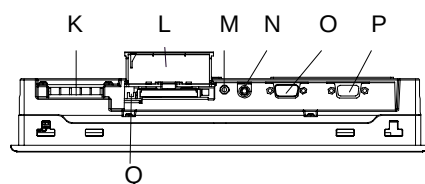
底面図
