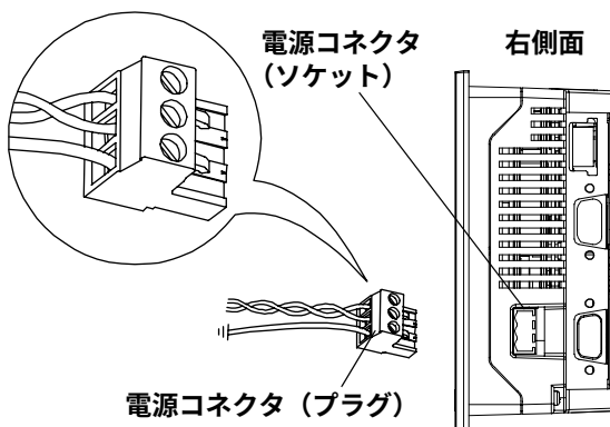
(図は GP-3300 シリーズ)
