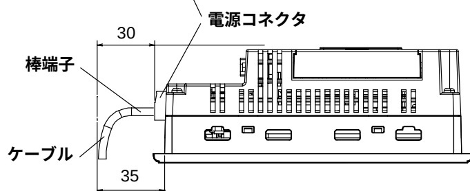
底面図
