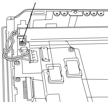
バックライトユニット固定ネジ
