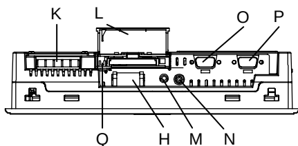
底面図 (AGP-35*0T)
