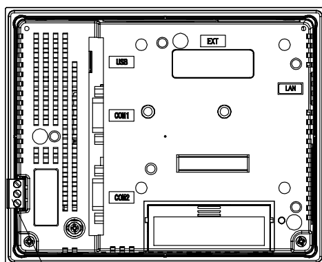
背面図
