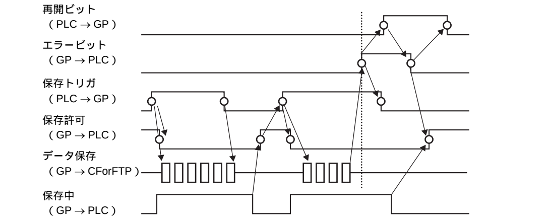
FTP 保存のタイミングチャート
