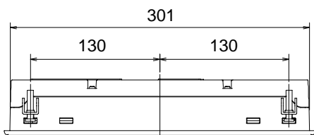
上面図
