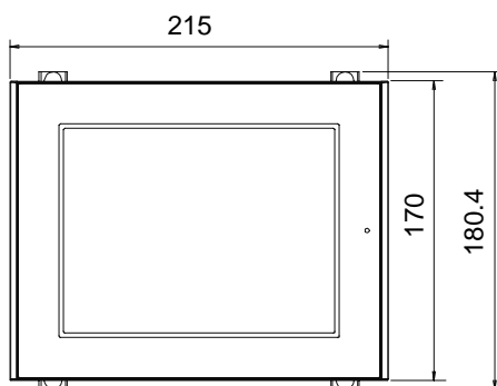
正面図
