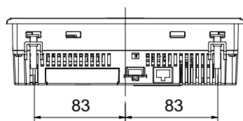
底面図
