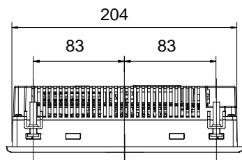
上面図
