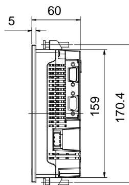
右側面図
