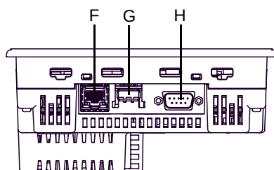
底面図
