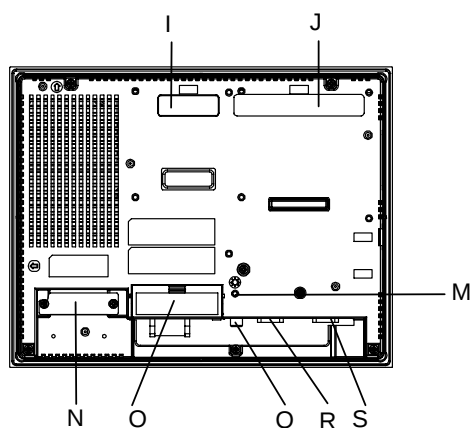
背面図 (AGP-35*0T)
