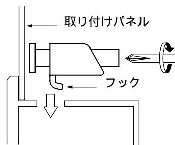
金具穴が上下にある場合 (図は GP-3300 シリーズ)
