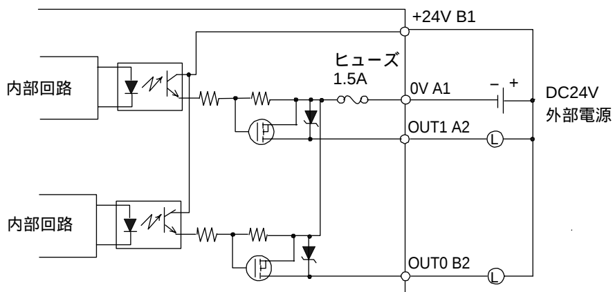
出力部回路 (シンクタイプ)
