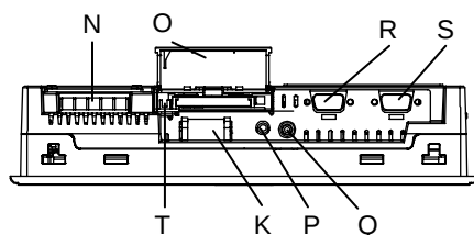
底面図 (AGP-35*0T)
