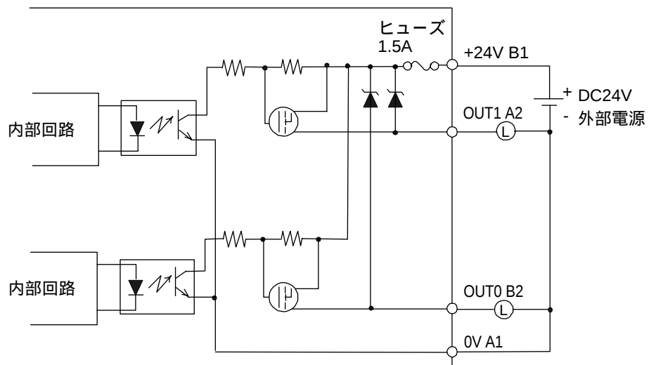
出力部回路 (ソースタイプ)
