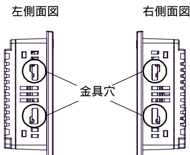
金具穴が左右にある場合 (図は GP-3200 シリーズ)
