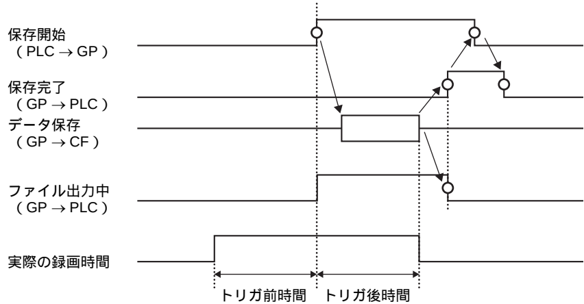
イベントレコーダのタイミングチャート
