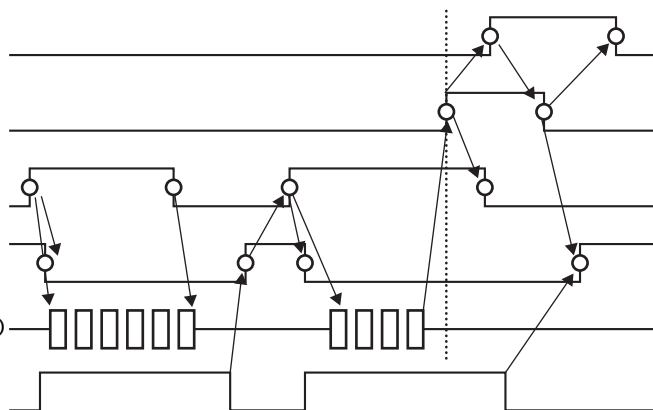
再開ビット (PLC → GP) エラービット (GP → PLC) 保存トリガ (PLC → GP) 保存許可 (GP → PLC) データ保存 (GP → CForP) 保存中 (GP → PLC)
