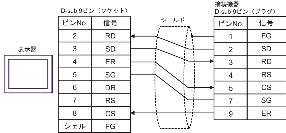
結線図 8
