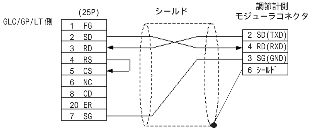
< 結線図 1 > 1:1 RS-232C
