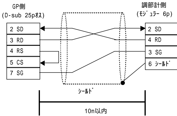
< 結線図 15 > RS-232C
