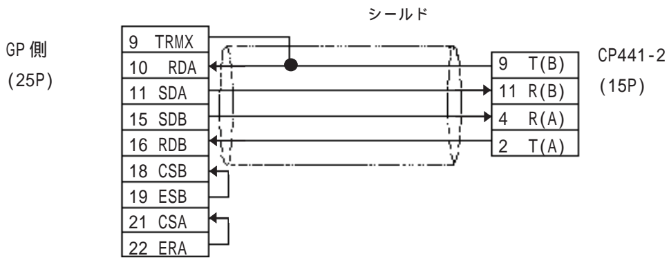
< 結線図 4 > RS-422
