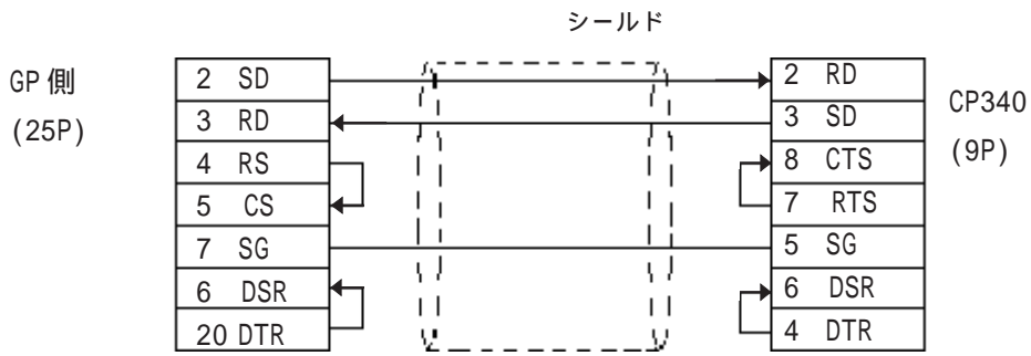
< 結線図 3 > RS-232C
