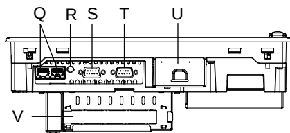
底面図 (PS-3650A シリーズ)
