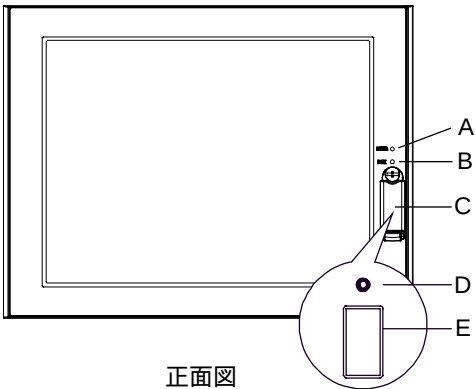
正面図 (PS-3650A/PS-3651A シリーズ共通)
