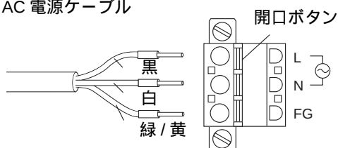
AC 電源ケーブル
