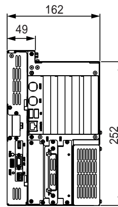
側面圖
