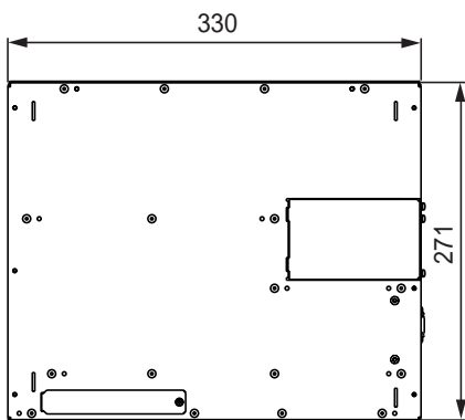
正面圖
