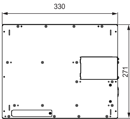
正面圖
