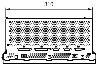
上面圖
