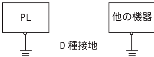
(a) 専用接地 最良
