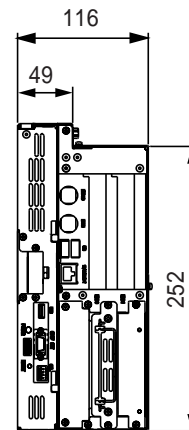
側面圖
