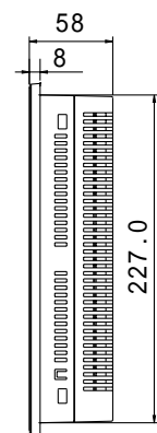
側面図
