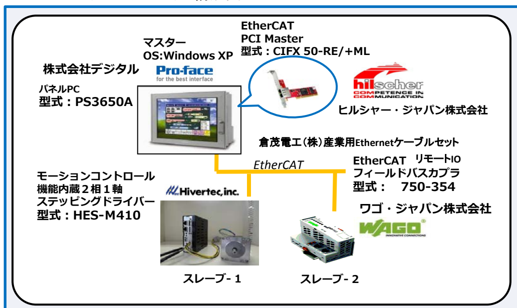
マルチベンダー・デモセット構成図
